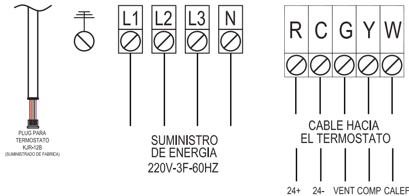
DIAGRAMA ELÉCTRICO PARA MODELO: IPCH300KF-5
